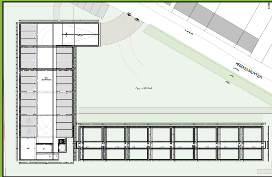
BOUWLAAG -1:
