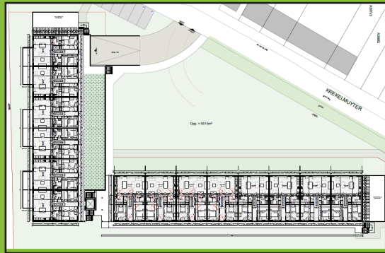
BOUWLAAG 0:
