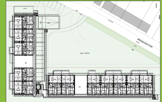
BOUWLAAG 1:
